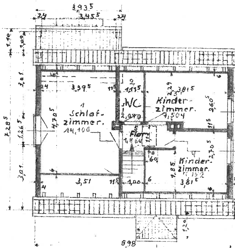
Dachgeschoss
