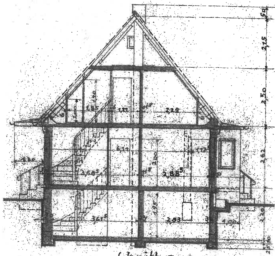
schnitt, a-a
