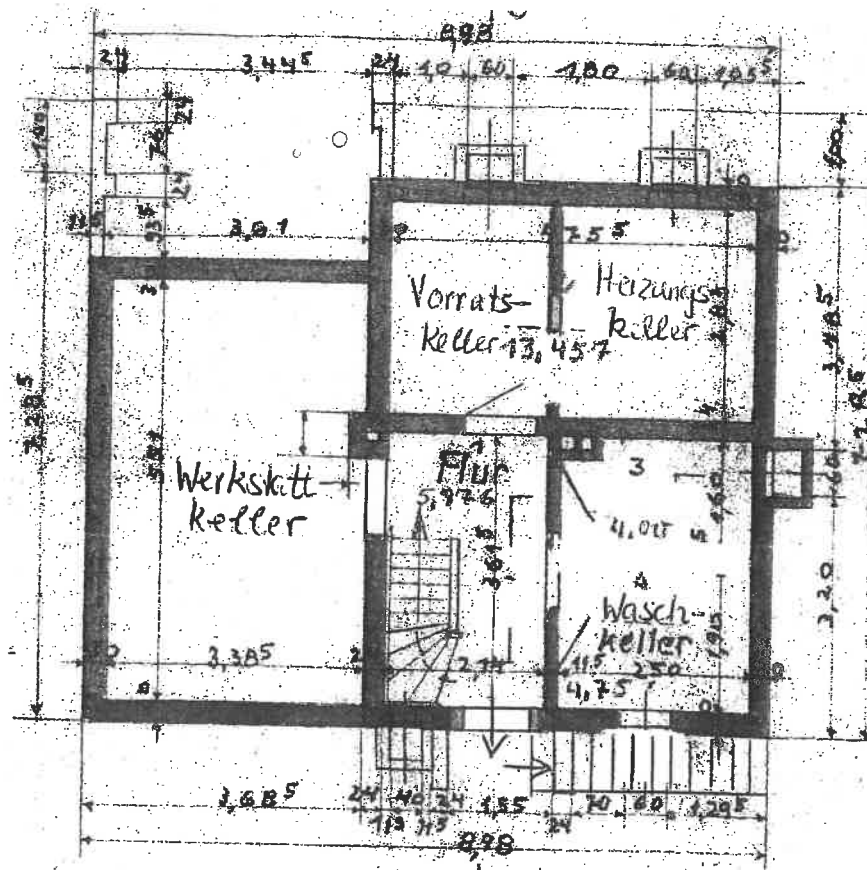
888 N Kellergeschoß
