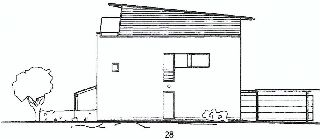
Giebelansicht
